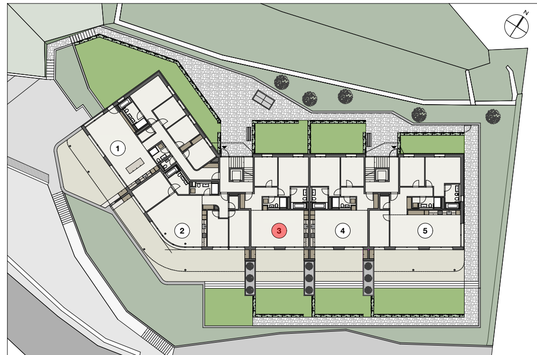
SITUATION REZ DE CHAUSÉE | 1:500
